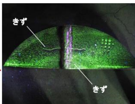
磁粉模様
